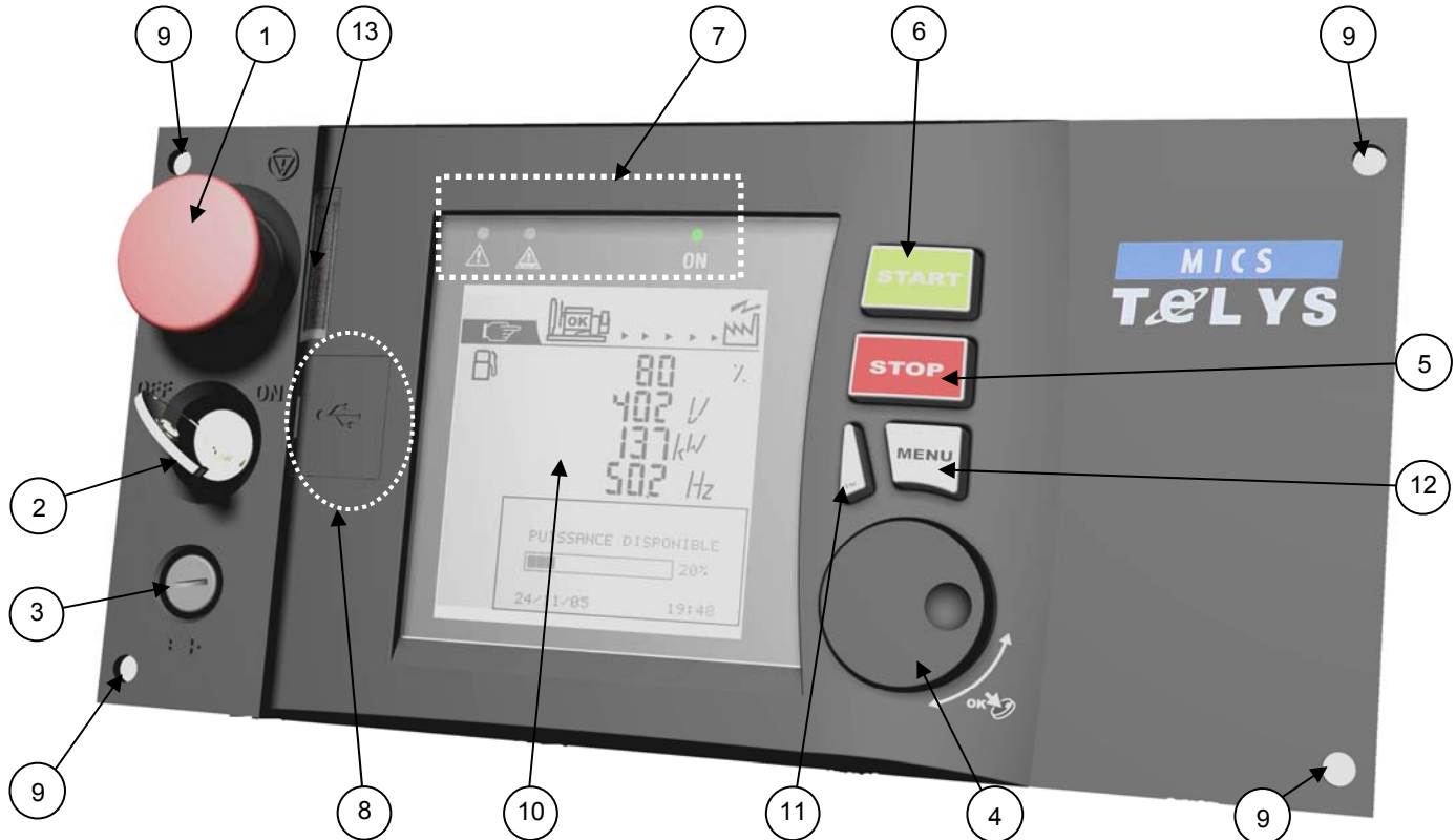
Bild 13: Översikt över kontrollpanelens framsida
